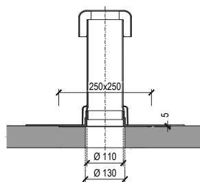
Вентиляционный выход DN 100
