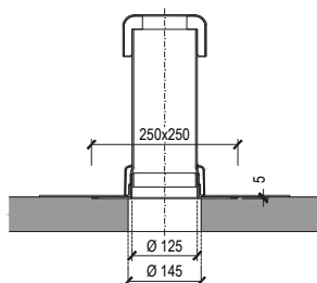
tetőre alkalmas szellőzőkürtőt DN 125
