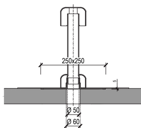
Вентиляционный выход DN 50
