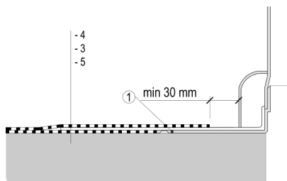
2. 2. b Detail napojení folie z asfaltových pásů
