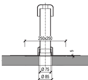
odvětrávací komínek DN 70
