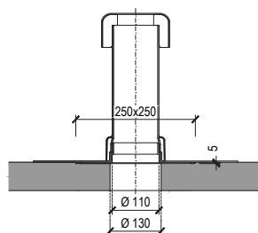
dachowy kominek odpowietrzający DN 100
