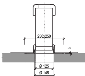
odvětrávací komínek DN 125
