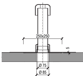
Вентиляционный выход DN 70
