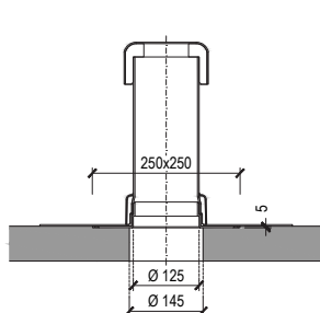
Вентиляционный выход DN 125
