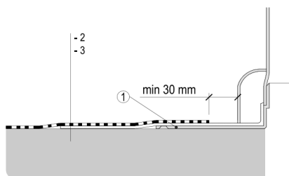
2. 2. a Alágyc PVC (TPO-FPO) fólia csatlakoztatásának részlete
