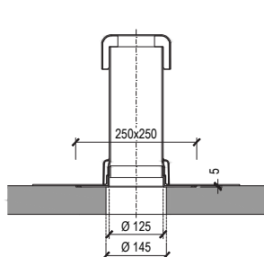
dachowy kominek odpowietrzający DN 125
