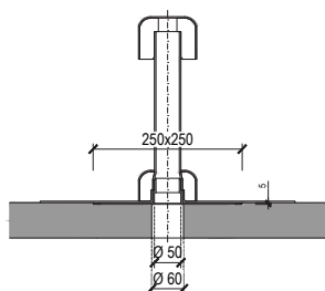
dachowy kominek odpowietrzający DN 50
