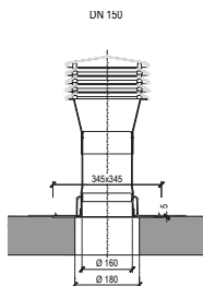
dachowy kominek odpowietrzający DN 150
