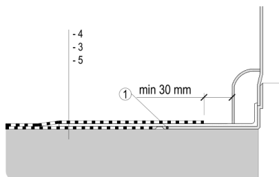
3.2b Узел крепления битумного материала
