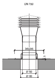
coș de aerisire pentru acoperiș DN 150
