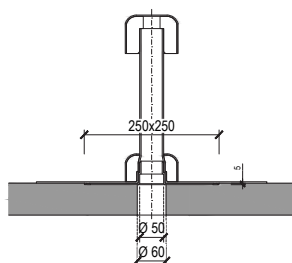
coș de aerisire pentru acoperiș DN 50
