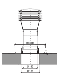
odvětrávací komínek DN 150
