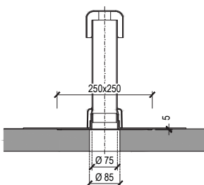
dachowy kominek odpowietrzający DN 70
