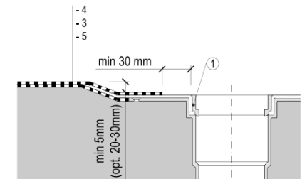
3.2.b Detail - Verbindungsfolie aus Bitumenstreifen
