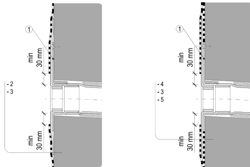
2.2.a Detail napojení folie mPVC (TPO-FPO)
