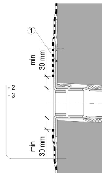
2.2.a Узел крепления ПВХ-мембраны (ТПО-ФПО)
