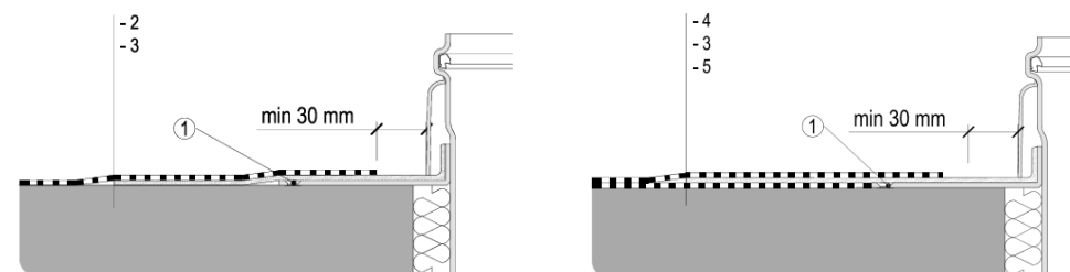
2.2.a Szczegół połączenia z folią mPVC (TPO-FPO)
