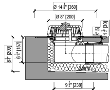
Desagüe de techo horizontal DN 4
